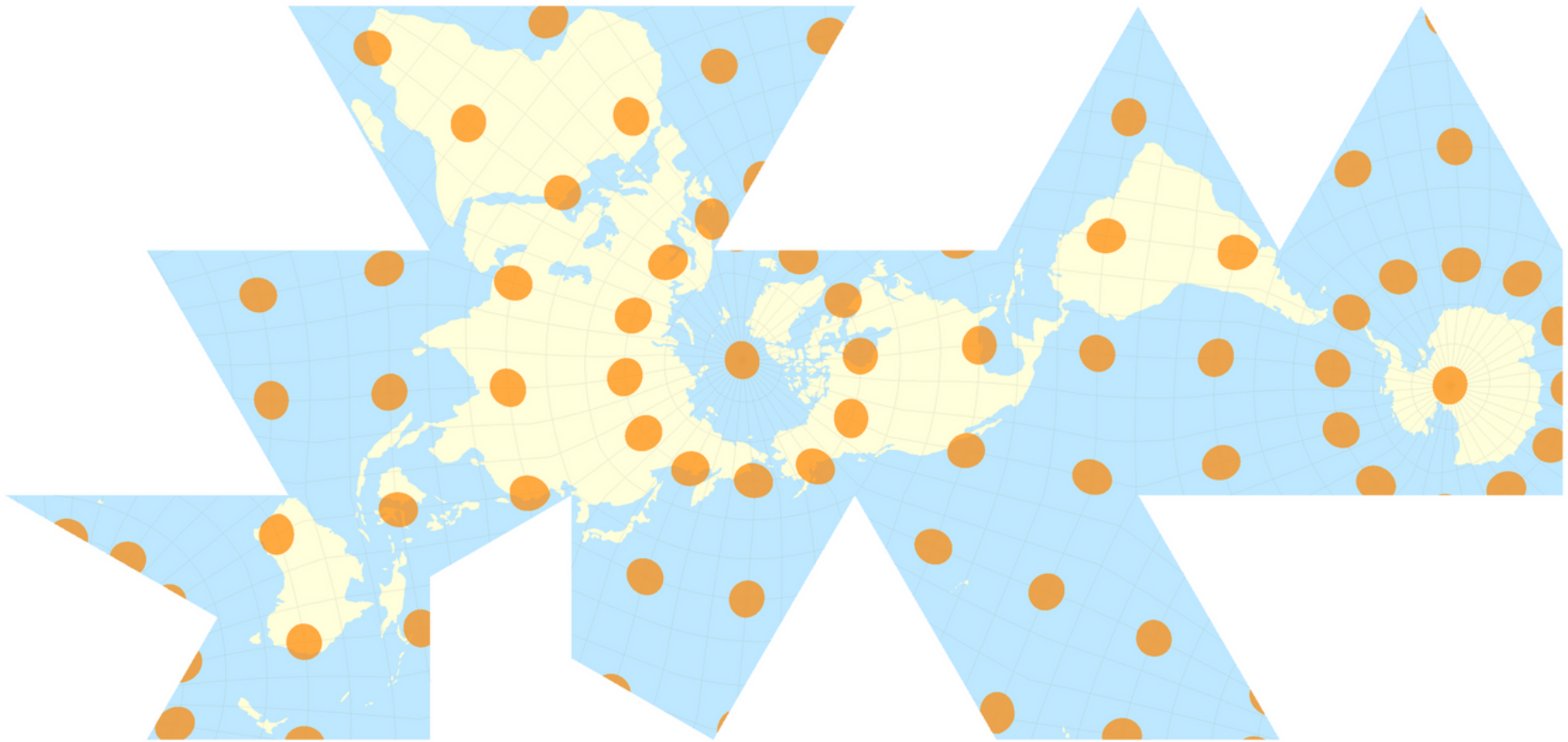
Carte du Monde avec indicateurs de Tissot pour représenter les déformations
